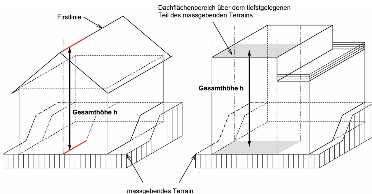
Figur 5.1 Gesamthöhe
