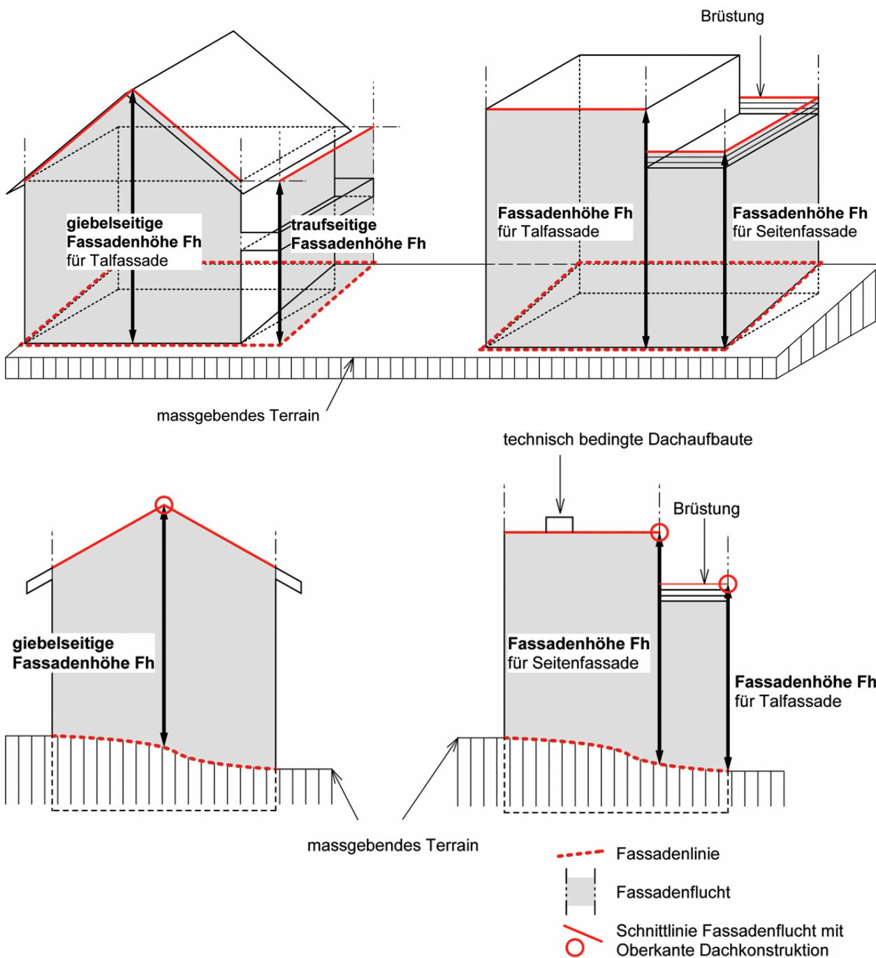
Figur 5.2 Fassadenhöhe
