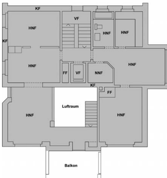
Grundriss 1. Obergeschoss:
